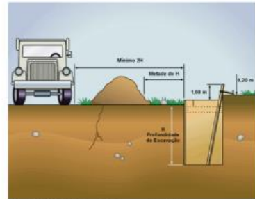
Figura 3 – Medidas de afastamento mínimo construídas adotadas
