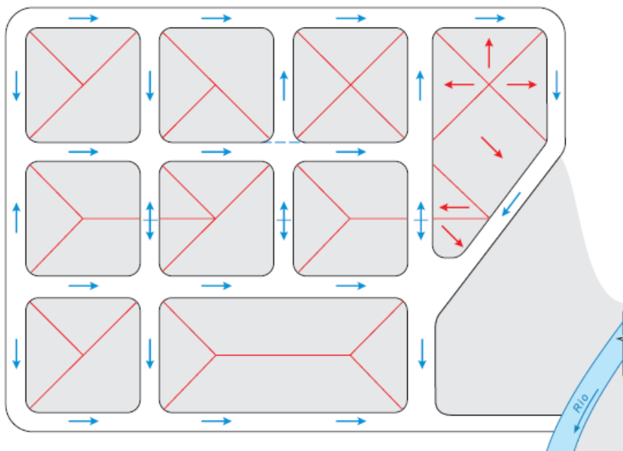
Figura 7 - Divisão de áreas de contribuição para as ruas (Fonte: Manual De Pavimentação Urbana, Diogo, Francisco José D'almeida, 2008).
